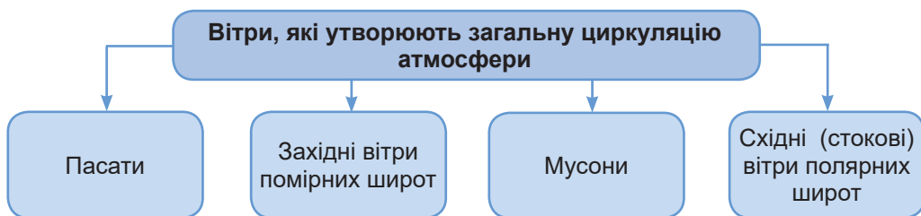
Мал. 41. Вітри, які визначають загальну циркуляцію атмосфери
