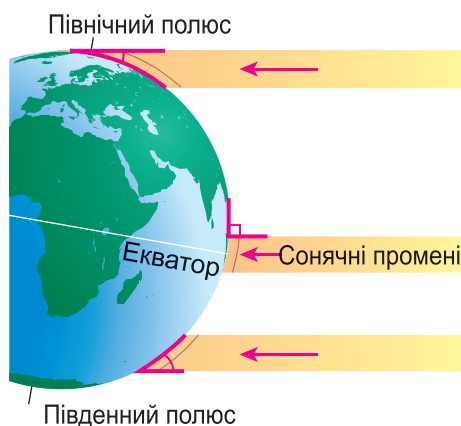
Мал. 35. Кут падіння сонячного проміння
