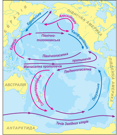
Мал. 190. Течії Тихого океану
