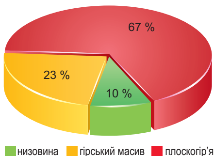
Мал. 54. Форми рельєфу Африки
