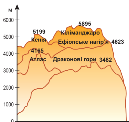
Мал. 55. Гірські масиви Африки
