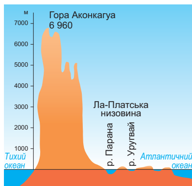
Мал. 98. Профіль рельєфу Південної Америки вздовж 32° пд. ш.
