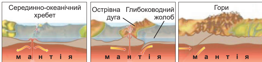
Мал. 31. Формування рельєфу поверхні Землі
