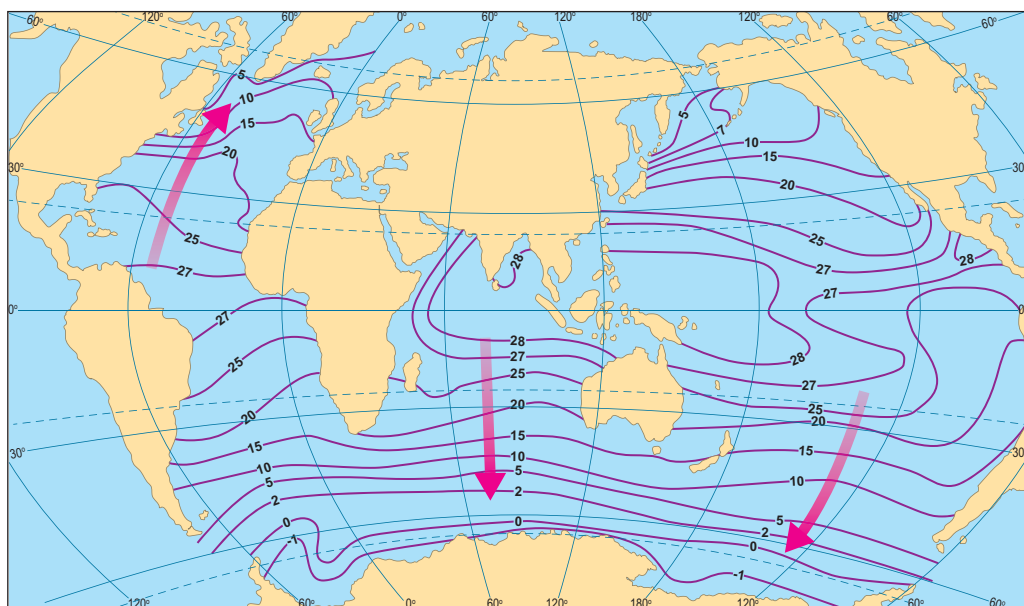
Мал. 36. Зміна середньорічної температури води на поверхні Світового океану
