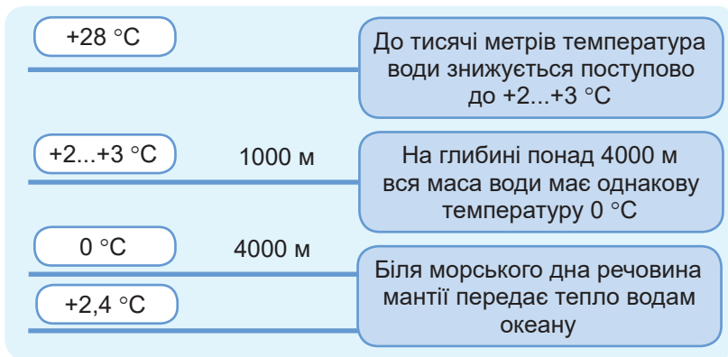
Мал. 37. Зміна температури води з глибиною
