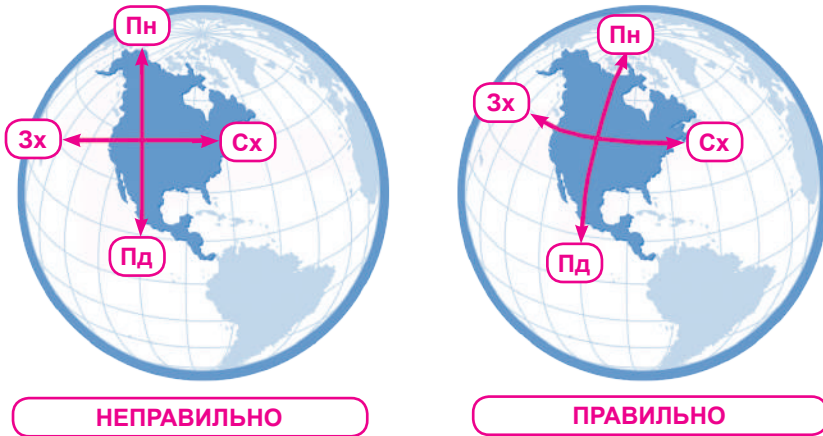
Мал. 17. Визначення напрямків за паралелями і меридіанами
