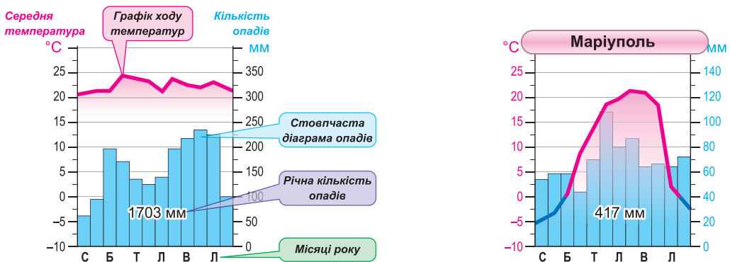
Мал. 44. Кліматична діаграма м. Маріуполя
