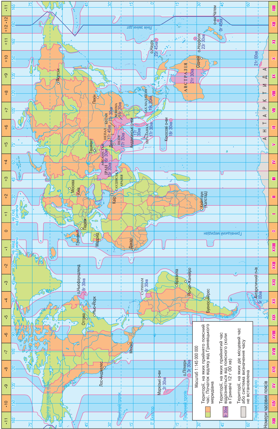
Мал. 7.2. Годинні пояси Землі
