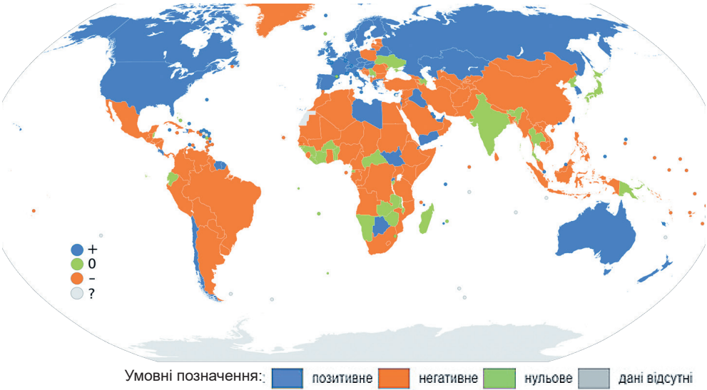
Мал. 21.3. Сальдо міграції у країнах світу
