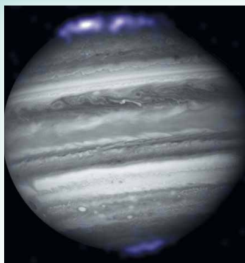
Мал. 3.20. Комбіноване фото Юпітера з телескопа «Габбл» та з рентгенівського телескопа «Чандра»
