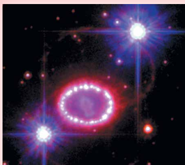
Мал. 5.11. Наднова SN 1987A зоря у Великій Магеллановій Хмарі (передає «Габбл» через 20 р. після вибуху зорі)
