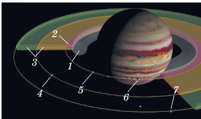
Мал. 3.21. Схема кілець Юпітера: 1 — гало, 2 — головне кільце, 3 — зовнішнє павутинне кільце, 4 — Амальтея, 5 — Адрастея, 6 — Метіда, 7 — Теба
