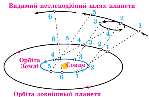
Мал. 1.14. Пояснення петлеподібного руху планет на основі теорії Коперника
