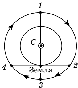
Мал. 1.16. Схема конфігурацій верхніх планет: 1 – сполучення; 2 – західна квадратура; 3 – протистояння; 4 – східна квадратура
