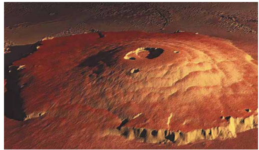
Мал. 3.16. Гора Олімп на Марсі
