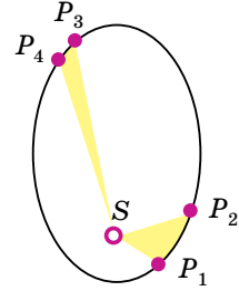
Мал. 1.26. Пояснення другого закону Кеплера
