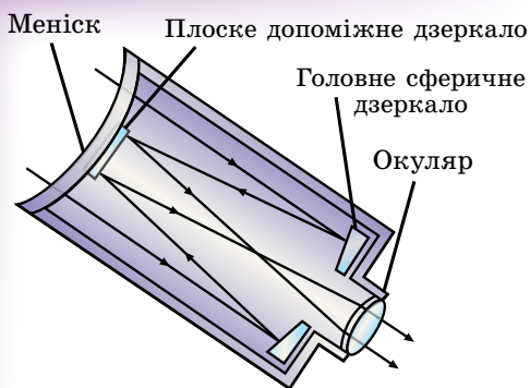
Мал. 2.6. Хід променів у дзеркально-лінзовому менісковому телескопі
