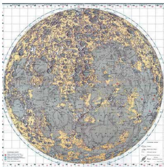
Мал. 3.4. Карта-схема 60-х рр. XX ст. найбільших деталей видимої в телескоп із Землі півкулі Місяця
