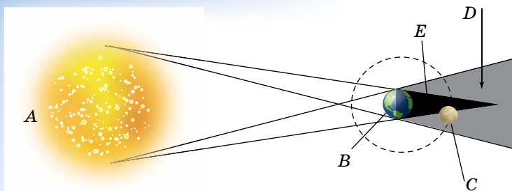
Мал. 1.23. Схема місячного затемнення. Розташування небесних тіл під час затемнення: A – Сонце; B – Земля; C – Місяць; D – напівтінь; E – повна тінь
