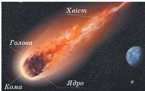
Мал. 3.42. Будова комети
