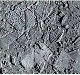
Мал. 3.30. Хаоси на супутнику Юпітера Європі
