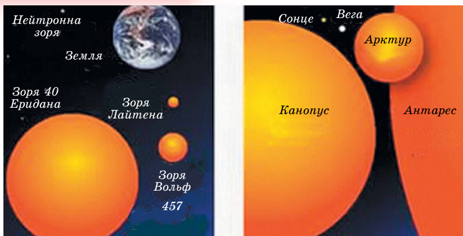
Мал. 5.4. Розміри деяких зір порівнянних з розмірами Землі (ліворуч) і Сонця (праворуч)
