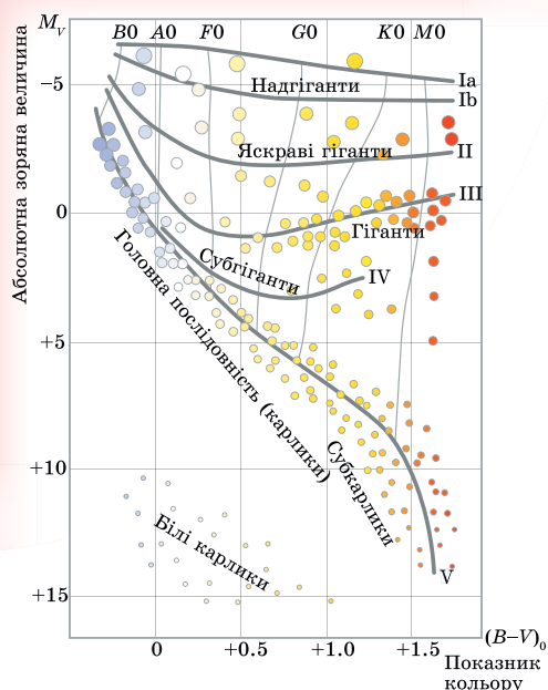
Мал. 5.6. Діаграма Герцшпрунга-Рассела
