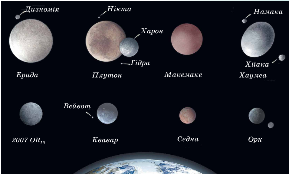
Мал. 3.37. Порівняльні розміри Землі та деяких карликових планет
