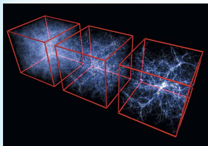
Мал. 7.14. Розподіл галактик у просторі
