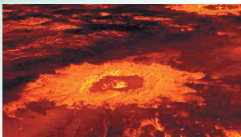
Мал. 3.11. Поверхня Венери
