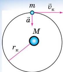
Мал. 1.31. Коловий рух тіл
