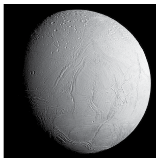
Мал. 3.36. Енцелад – супутник Сатурна. Фото «Кассіні–Гюйгенс» (2005 р.)
