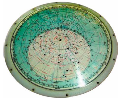
Мал. 1.32. Рухома карта зоряного неба
