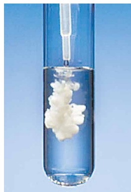
Рис. 32.2. Білий дрібнокристалічний осад барій сульфату – зовнішній ефект якісної реакції на катіони Барію
