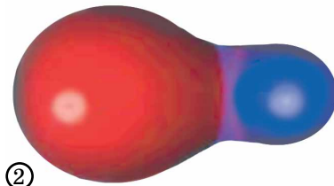
Рис. 6.1. 1. Масштабна модель молекули води. 2. Схематичне зображення диполя
