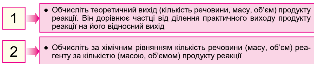
Рис. 13.3. Алгоритм обчислення кількості (маси, об'єму) реагенту, якщо відомі кількість (маса, об'єм) продукту реакції та його відносний вихід
