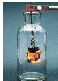
Рис. 19.4. Окиснення міді в атмосфері кисню
