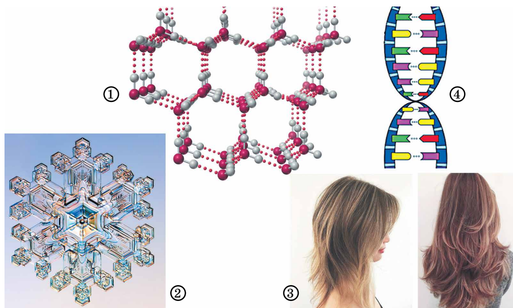
Рис. 6.6. Багатоликий водневий зв'язок. 1. Водневі зв'язки в кристалічній структурі льоду. 2. Сніжинки складаються з кристаликів льоду (висловте припущення, чому в будь-якої сніжинки саме шість променів). 3. Завивання та розпрямлення волосся під дією високої температури послаблює водневі зв'язки між молекулами білка, тому волосся змінює форму, однак швидко воно намокає, то повертається до початкового стану. 4. У подвійній спіралі молекули ДНК нітрогеновмісні основи одного з ланцюгів сполучені з нітрогеновмісними основами іншого ланцюга водневими зв'язками згідно з принципом комплементарності: аденін з'єднується лише з тиміном, гуанін – лише із цитозином
