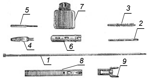
Приладдя для обслуговування автомата
