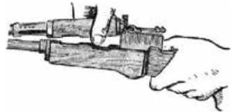
9. Відокремити газову трубку зі ствольною накладкою
