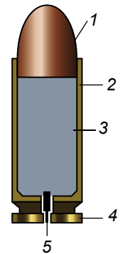
Будова унітарного патрона: 1 – куля; 2 – гільза; 3 – порох; 4 – фланець (закраїна); 5 – капсуль
