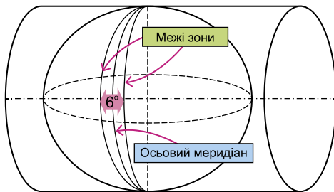
Проекція Гауса–Крюгера
